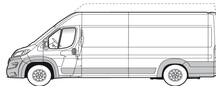
L4 (RADSTAND 4.035 mm – MIT VERLÄNGERTEM ÜBERHANG | FAHRZEUGLÄNGE / FAHRZEUGBREITE: 6363 / 2.100 mm
